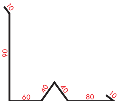
Lišta boční se stojatou drážkou r.š. 333 mm č. 3
