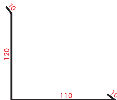
Lišta boční plochá r.š. 250 mm č. 4
