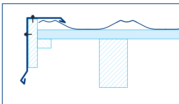
Závětrná lišta horní
