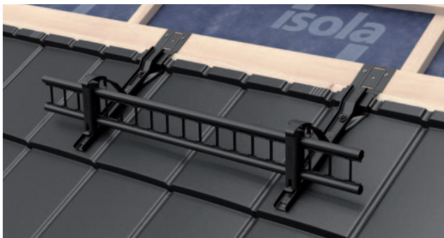
Bezpečnostní systém TopSec – systém sněhové zábrany
